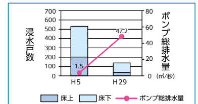
大野川直轄管理区間のポンプ排水量と浸水被害の推移
