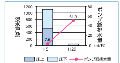
大分川直轄管理区間のポンプ排水量と浸水被害の推移
