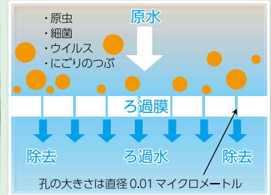
膜モジュール
