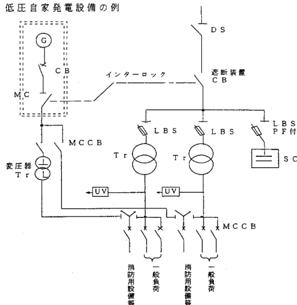
低圧自家発電設備の例
