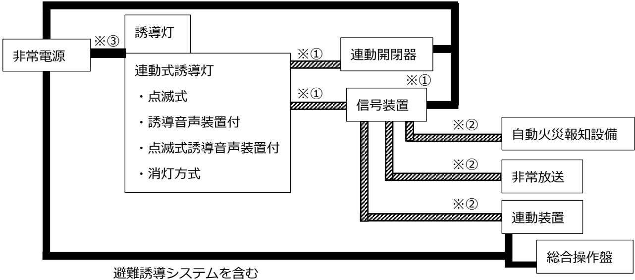
避難誘導システムを含む
