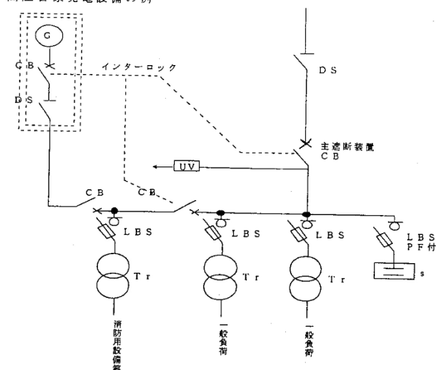
高圧自家発電設備の例
