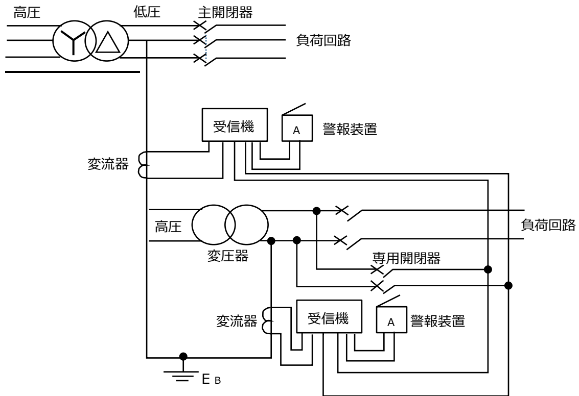
例 3 変圧器の二次側定圧電路に接続された接地線に設ける方式の場合
