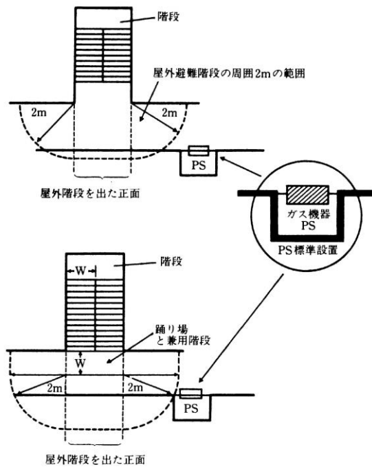
図1 屋外階段を出た正面又は屋外避難階段の周囲2mを避けた設置例
