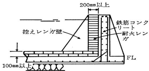
図5 砂床型設置の例
