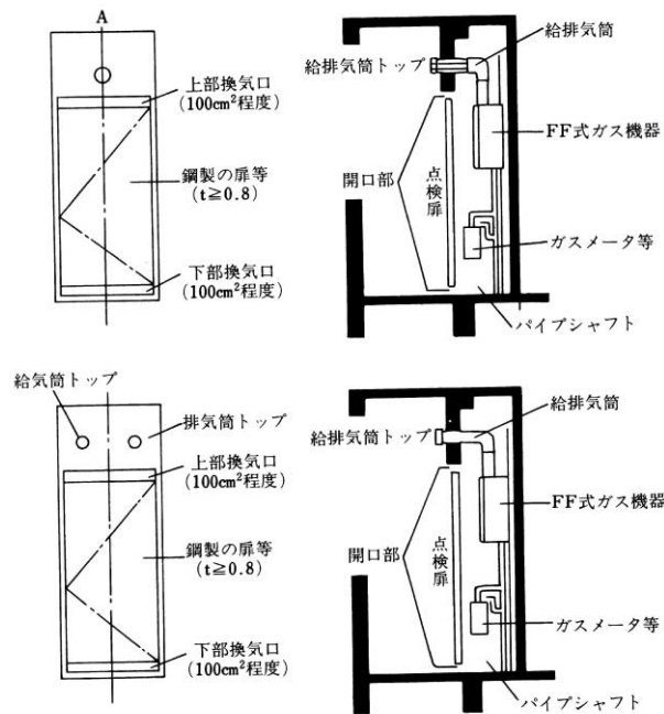
図 10 パイプシャフト等の扉に設ける開口部の例
