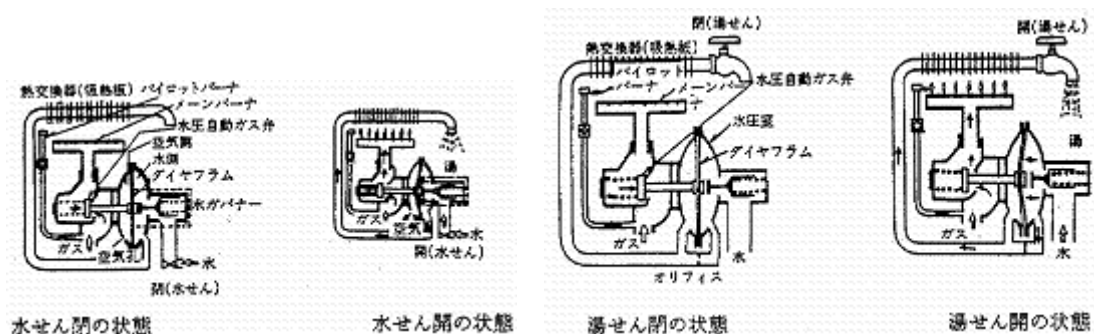
図2 ガス瞬間湯沸器の作動原理の例
