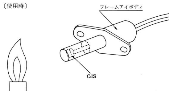
図8 点火安全装置の例（フレイムアイによるもの）
