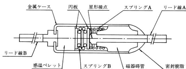
過熱防止装置の例（温度ヒューズによるもの）
