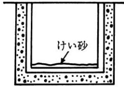
図3 ピット型の設置例
