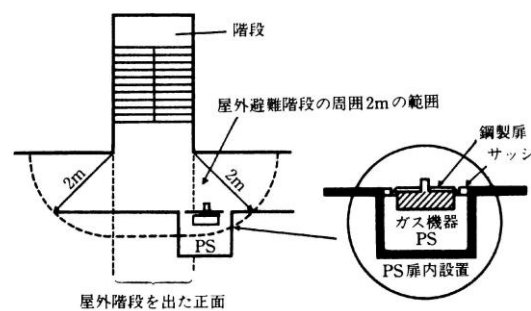
図2 屋外階段を出た正面又は屋外避難階段の周囲2mの範囲内への設置例
