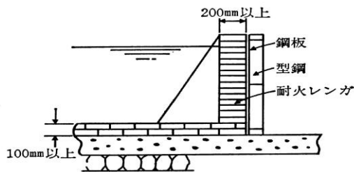
図6 堰堤型設置の例
