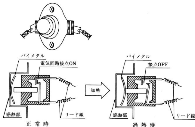
図9 過熱防止装置の例（バイメタルによるもの）
