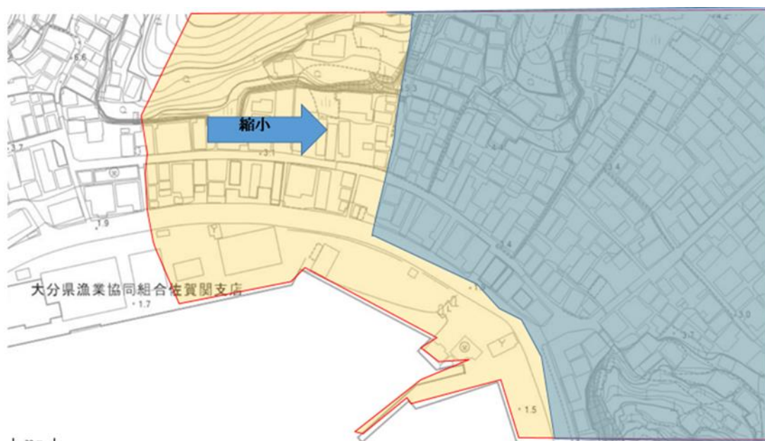
消防警戒区域図(西端詳細)
