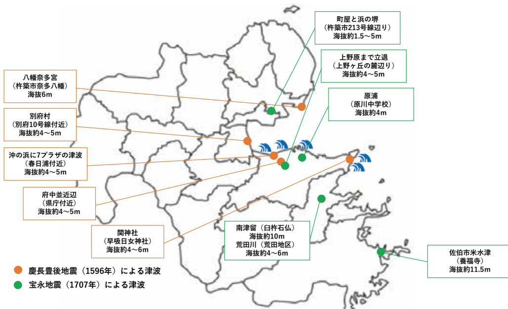
【出典：大分県HP（歴史古文書における慶長豊後地震及び宝永地震の津波被害箇所と津波高）引用編集】
