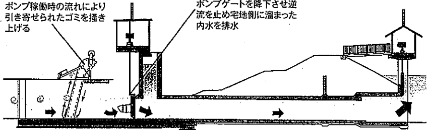
ゲート式ポンプ イメージ図
