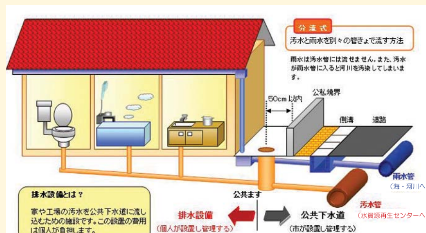
排水設備のしくみ（大分市下水道部資料）
