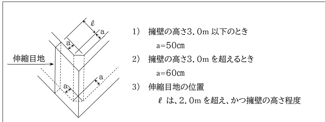
図 2-26 隅角部の補強方法および伸縮目地の位置
