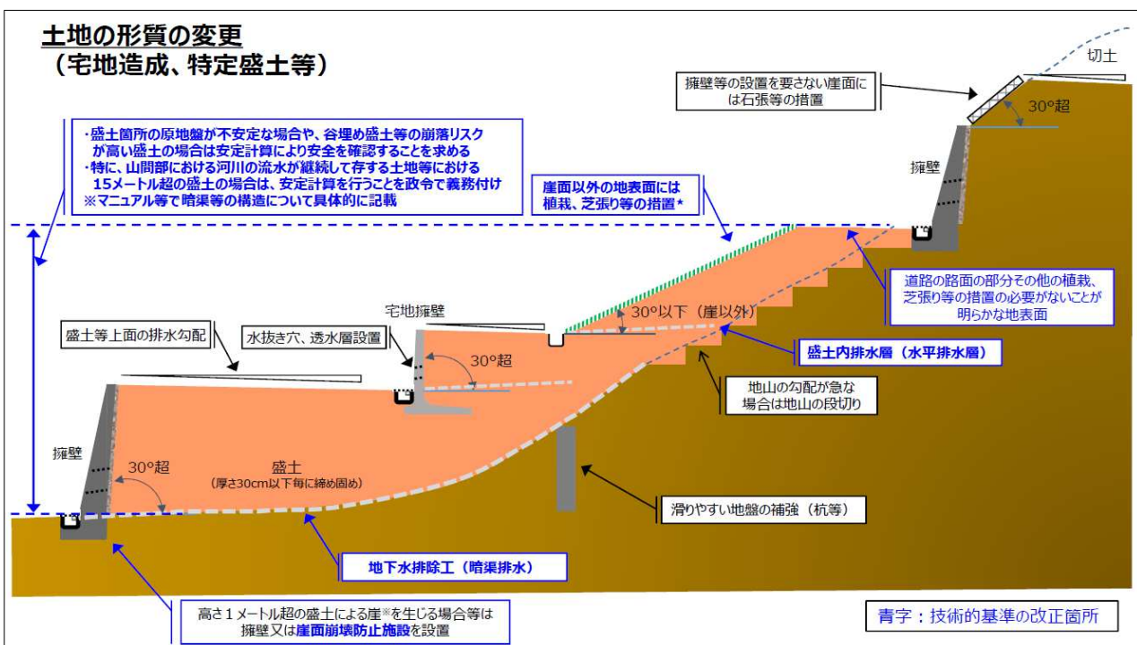
図 2-1 土地の形質の変更に係る技術的基準(政令)全般の概念図
