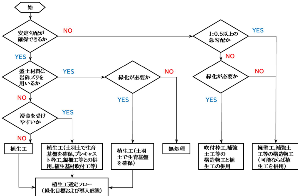
図 2-30 盛土法面における法面保護選定フロー
