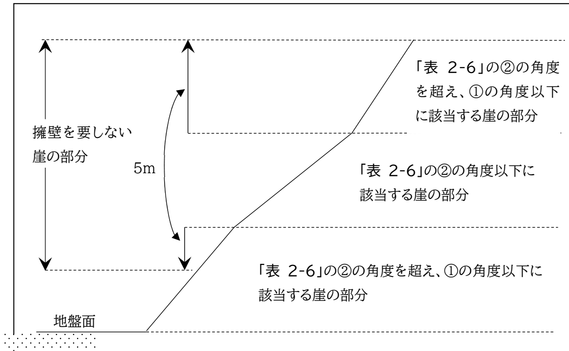
図 2-16 擁壁を要しない崖または崖の部分 『盛土等防災マニュアルの解説』(盛土等防災研究会)
