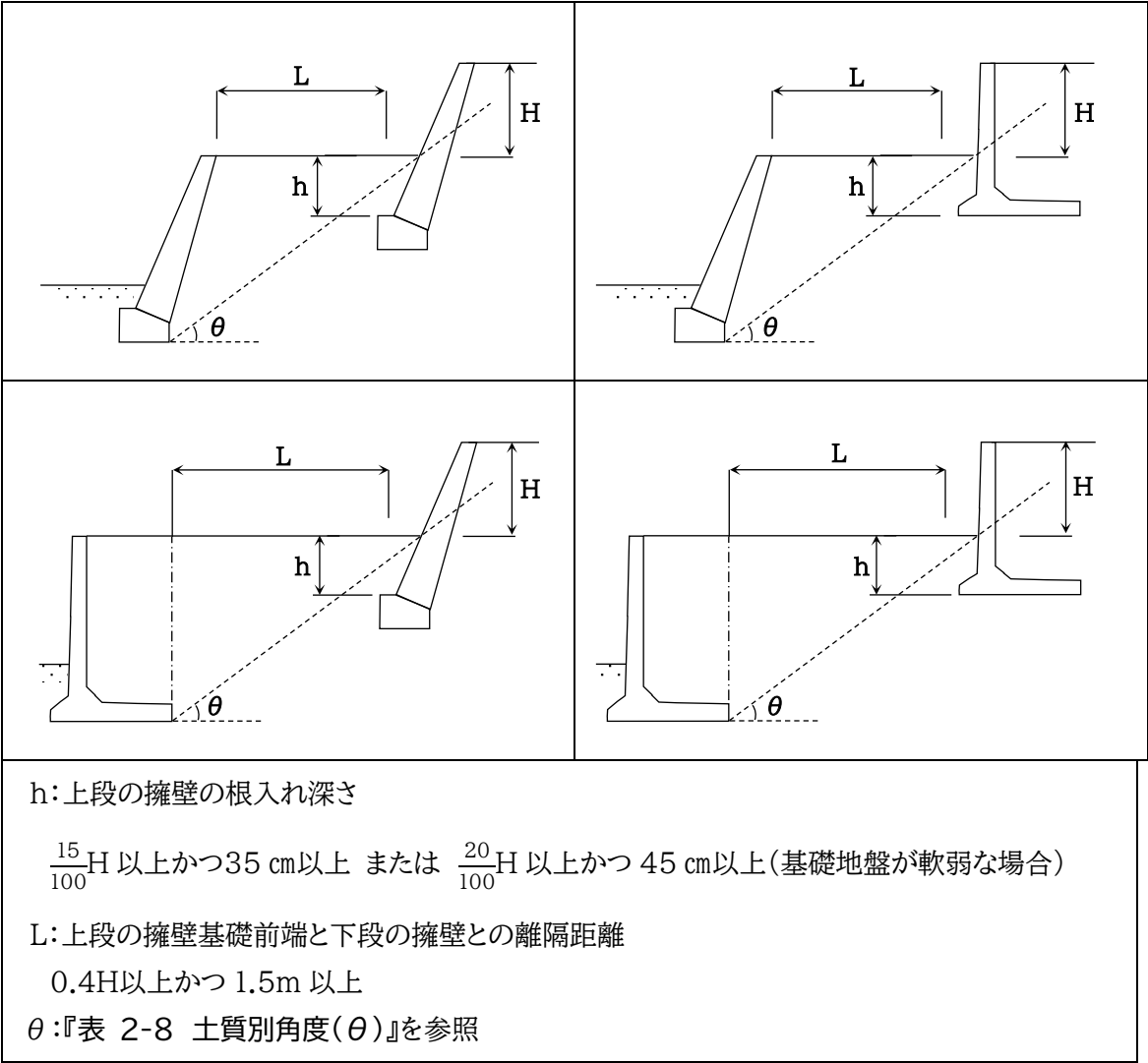
図 2-24 上部・下部擁壁を近接して設置する場合
