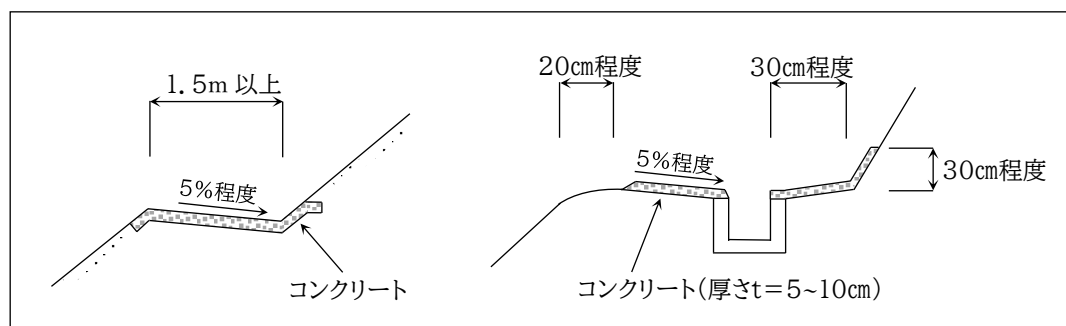
図 2-32 法面小段排水工
