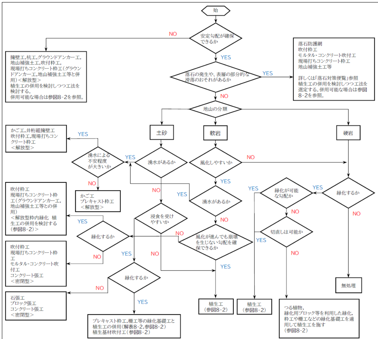
図 2-29 切土法面における法面保護工選定フロー 『道路土工－切土工・斜面安定工指針』(社)日本道路協会
