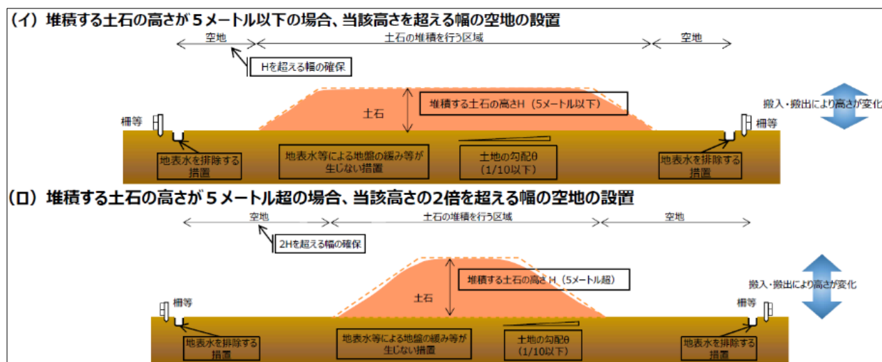
図 2-34 土石の堆積に係る技術的基準(政令)全般の概念図
