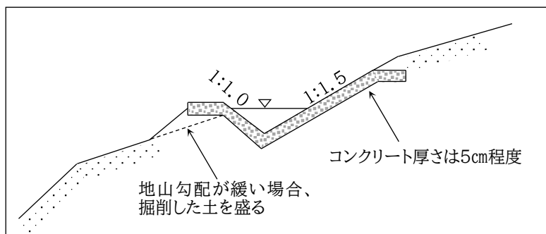
図 2-31 法肩排水工(コンクリート等による排水工)
