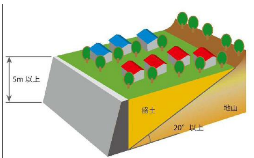
図 2-10 腹付け型大規模盛土造成地
