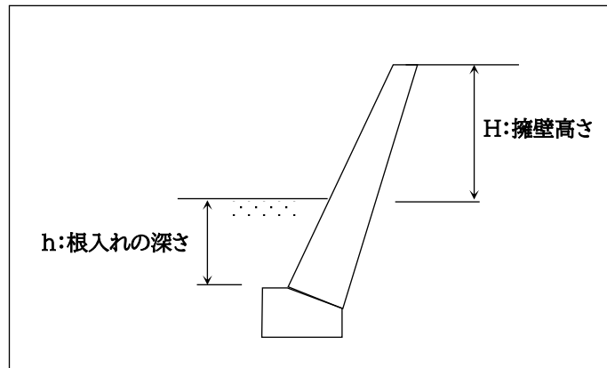
図 2-19 根入れの深さ(令第 10 条第4号)
