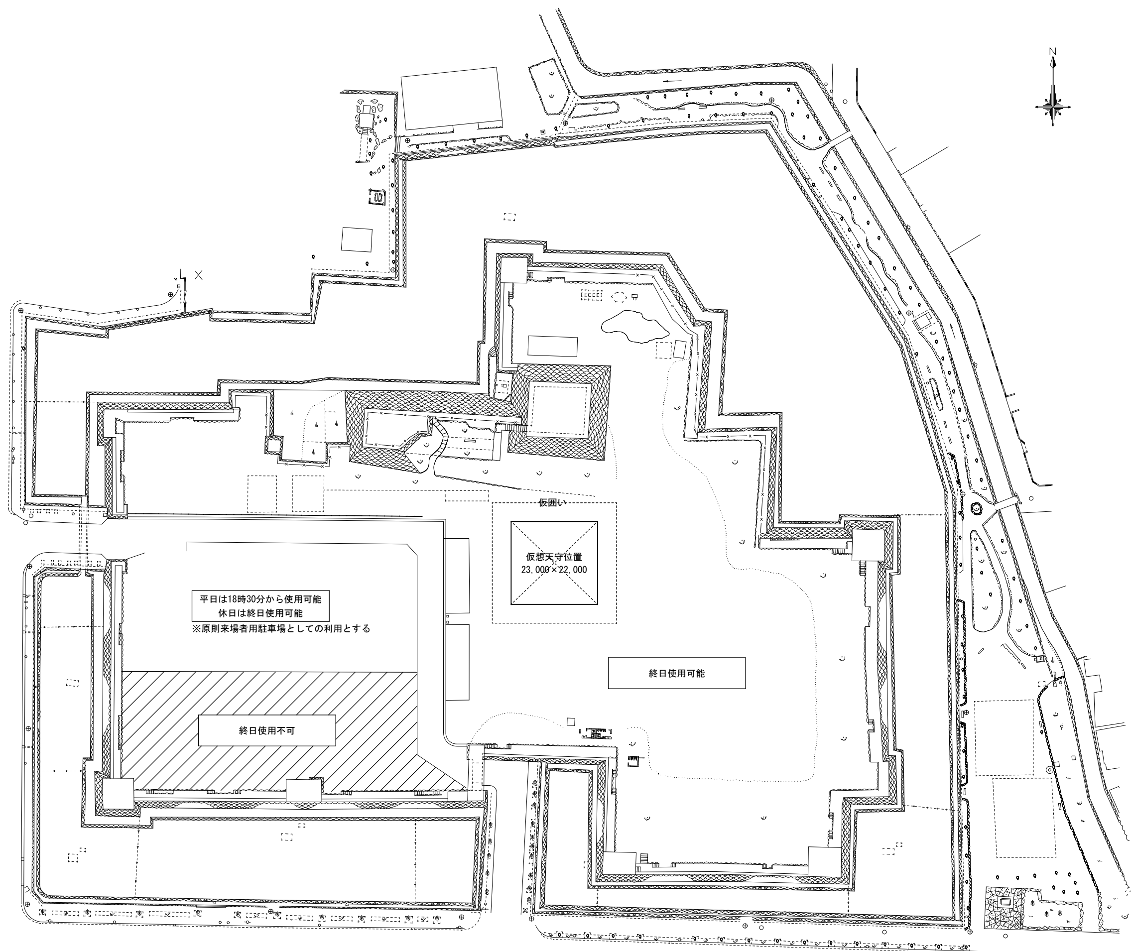
配置図 S=1/1,000
