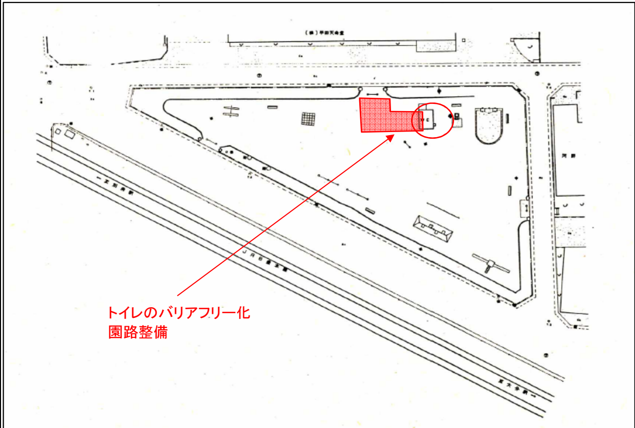
田室公園計画平面図
