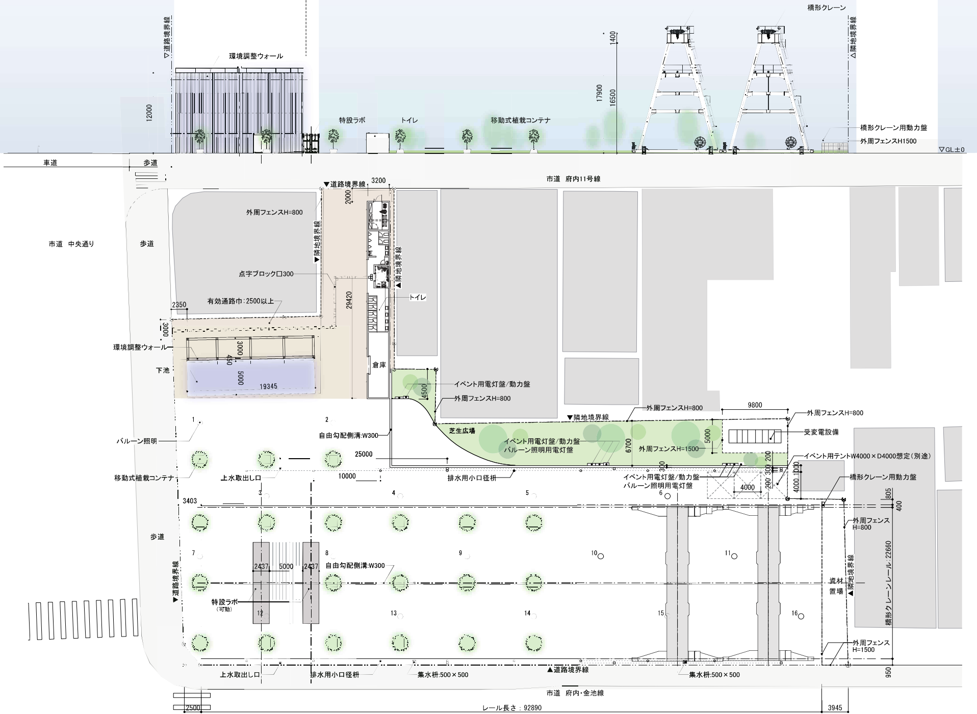
平面図・立面図 1/400 (A3)
