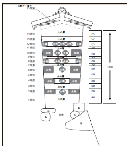
▲復旧土塀断面図
