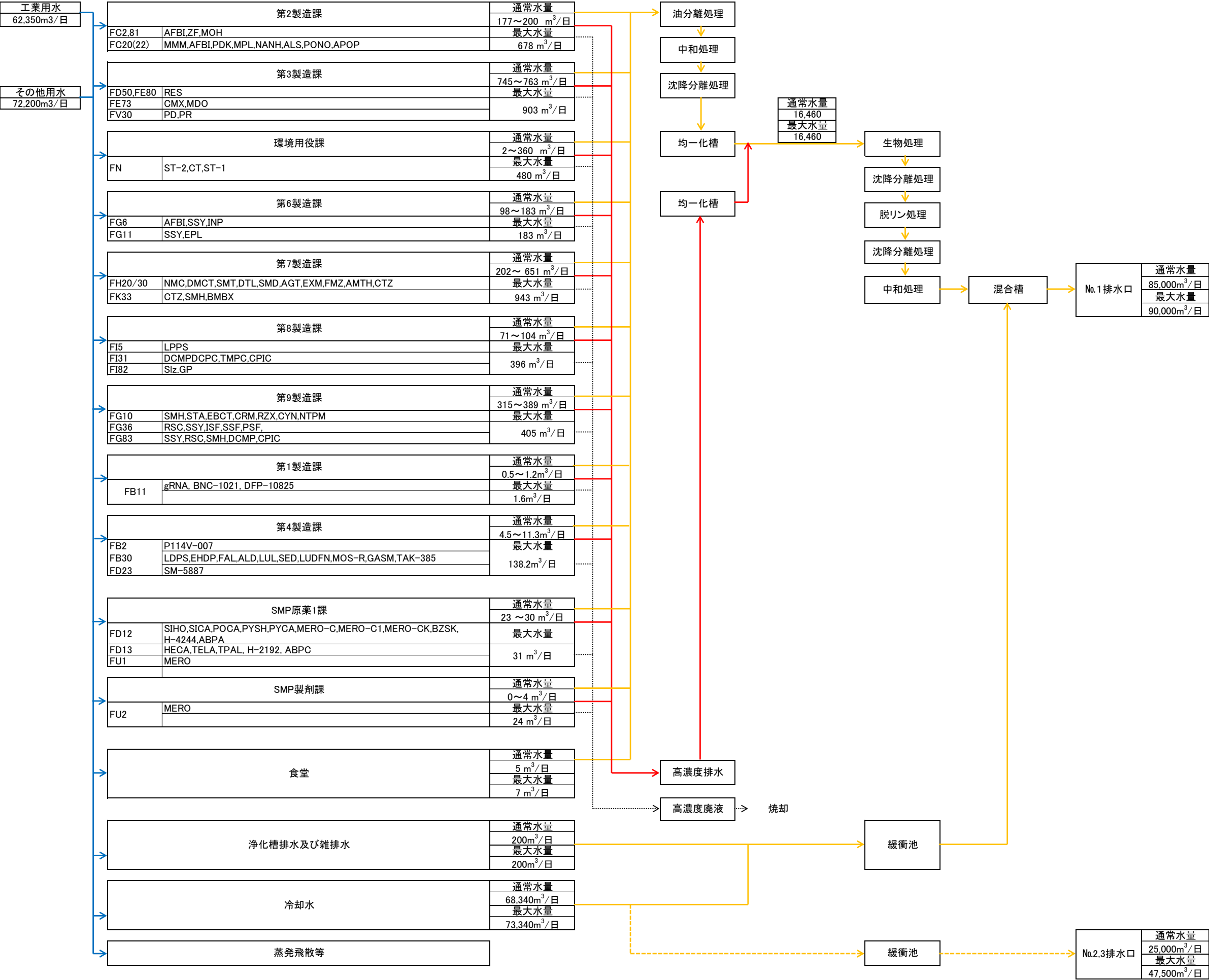
廃水処理系統図
