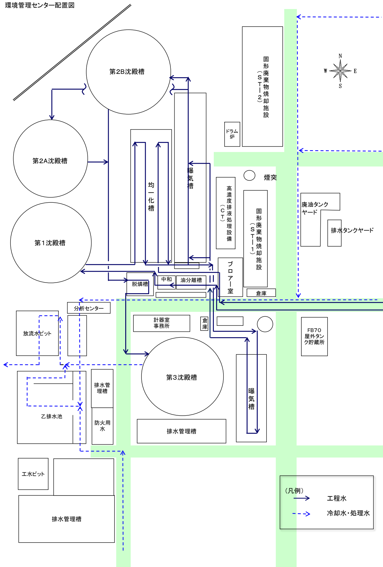
環境管理センター配置図
