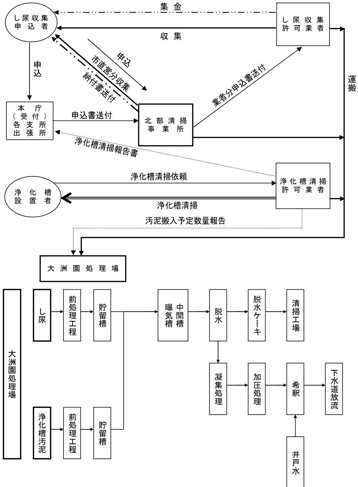
図2-1 収集運搬・処理体系図（大分地区・佐賀関地区）
