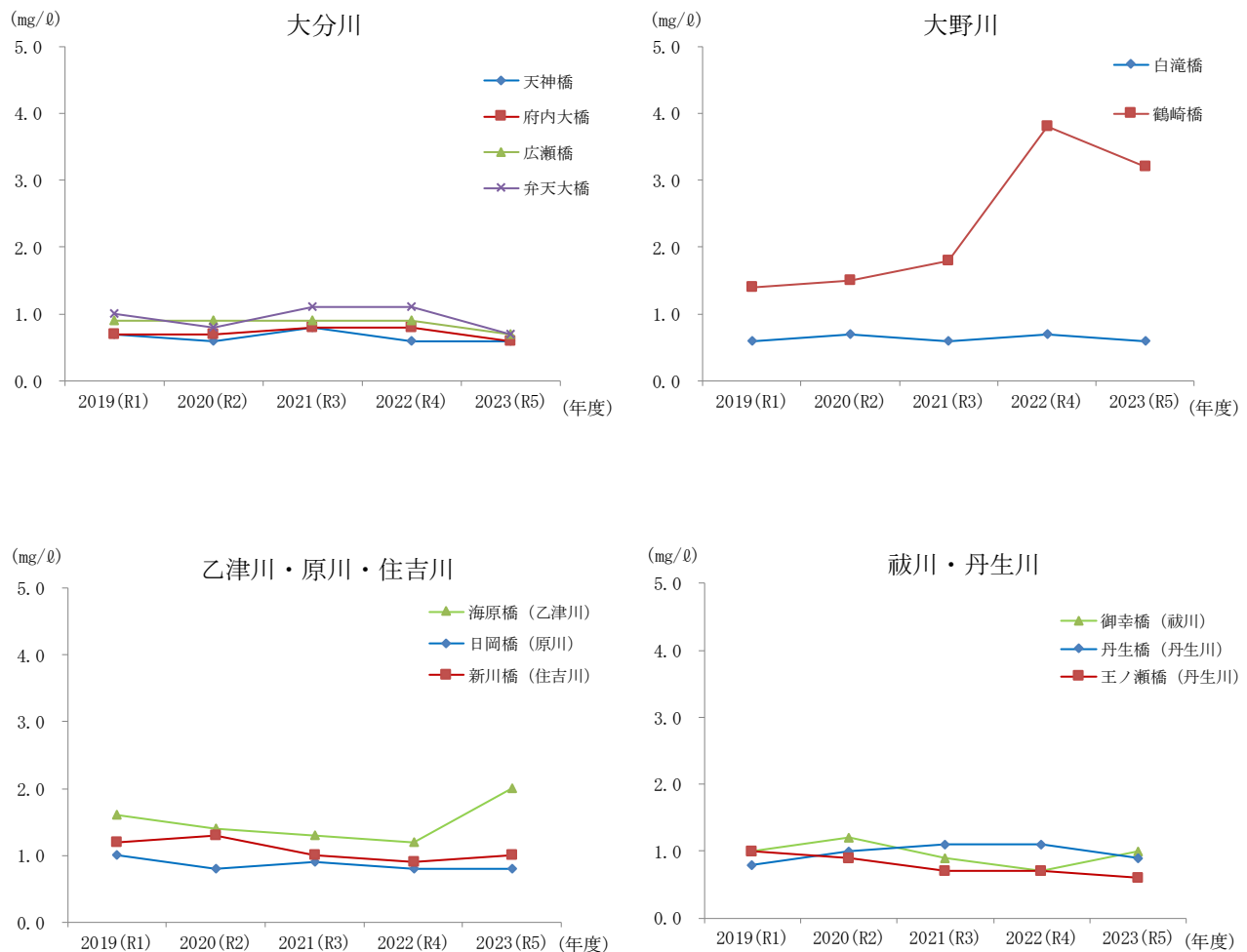
資 6－9 河川の環境基準点におけるBOD年平均値の経年変化
