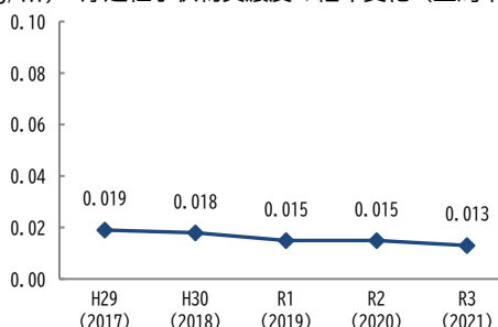
(mg/m 3 ) 浮遊粒子状物質濃度の経年変化（全局平均値）
