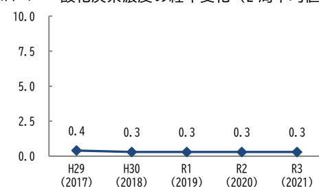
(ppm) 一酸化炭素濃度の経年変化 (2局平均値)
