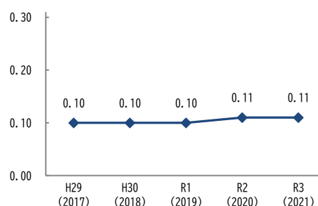
(ppmC) 非メタン炭化水素濃度の経年変化 (全局平均値)
