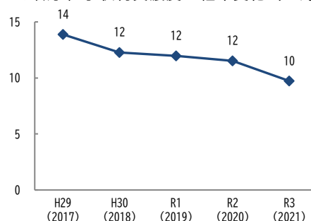
( \mu\text{g}/\text{m}^3 ) 微小粒子状物質濃度の経年変化 (全局平均値)
