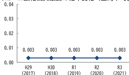
(ppm) 二酸化窒素濃度の経年変化（全局平均値）
