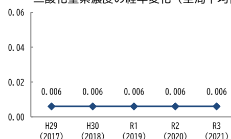
(ppm) 光化学オキシダント濃度の経年変化（全局平均値）
