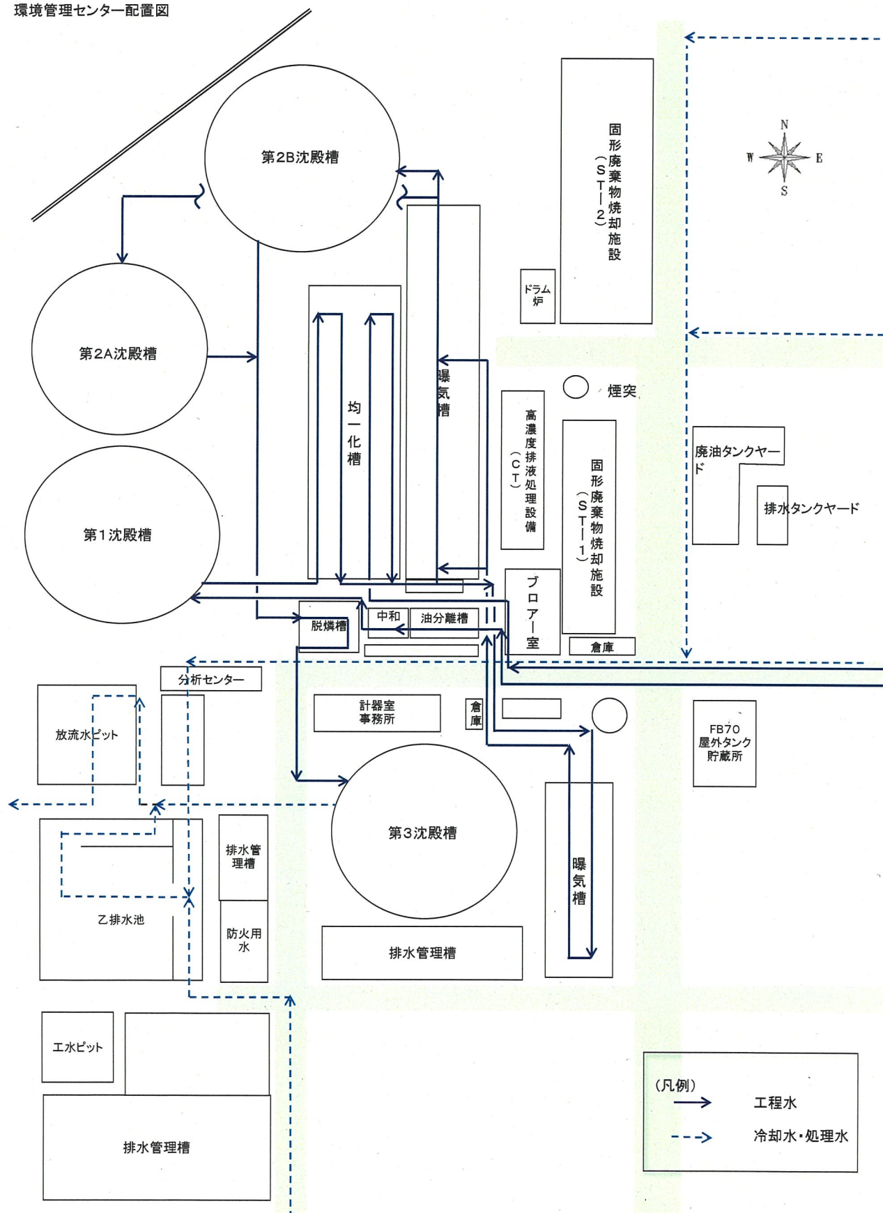
環境管理センター配置図
