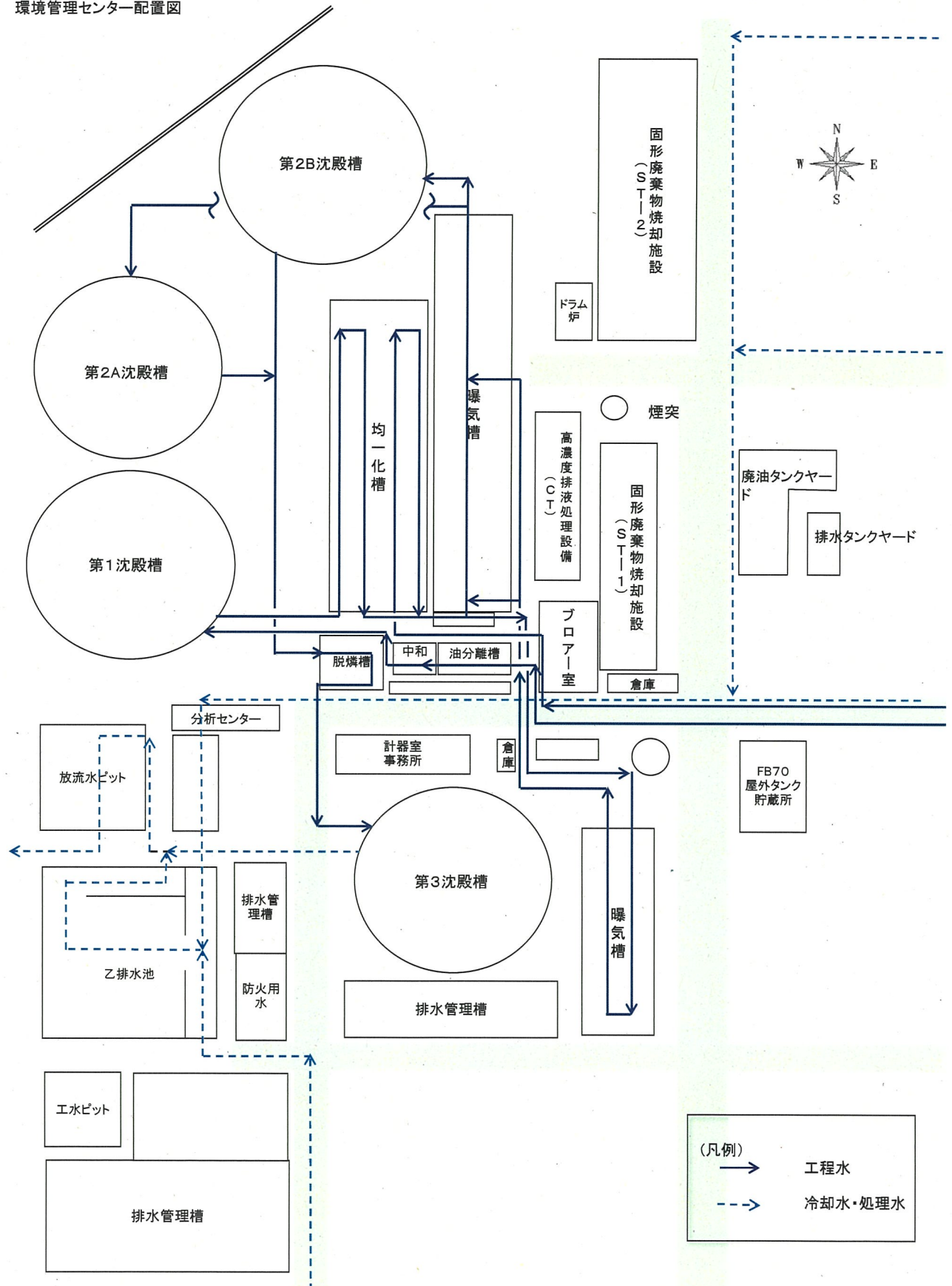
環境管理センター配置図
