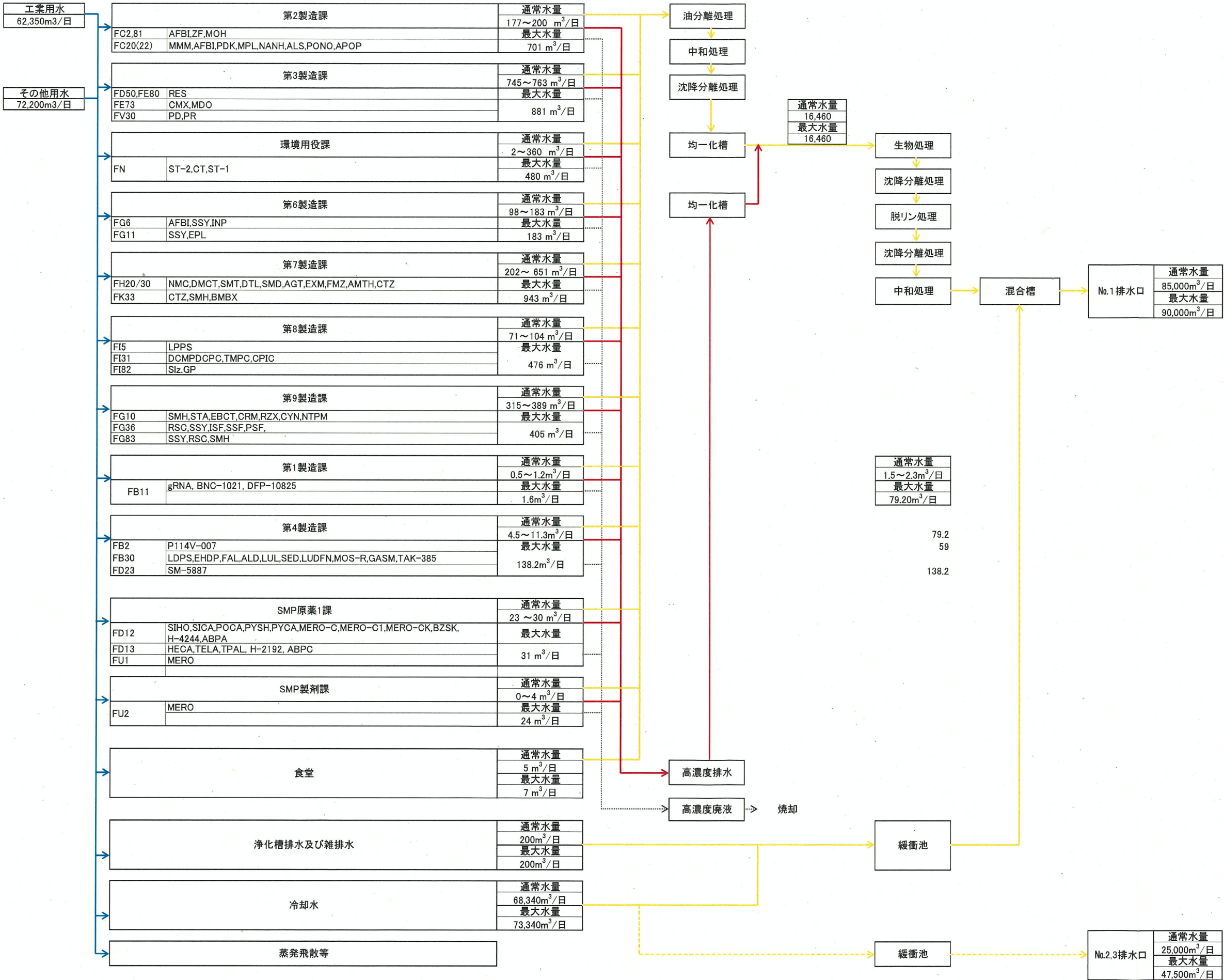
廃水処理系統図
