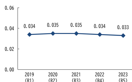
(ppm) 一酸化炭素濃度の経年変化（平均値）
