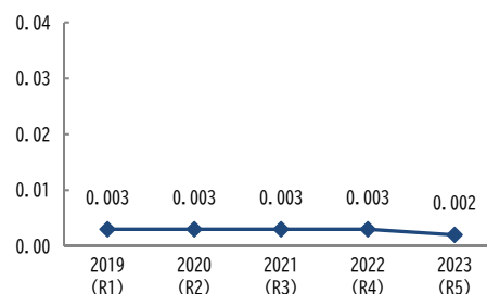
(ppm) 二酸化窒素濃度の経年変化（全局平均値）
