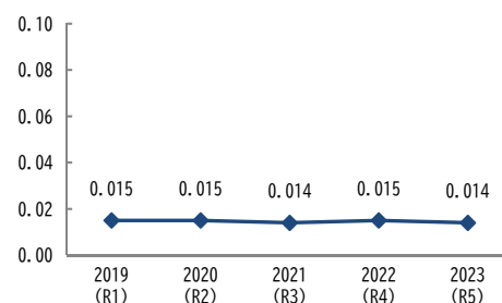
( \text{mg}/\text{m}^3 ) 浮遊粒子状物質濃度の経年変化（2局平均値）
