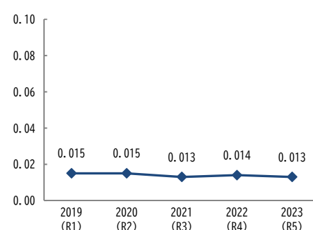
(mg/m³) 浮遊粒子状物質濃度の経年変化（全局平均値）
