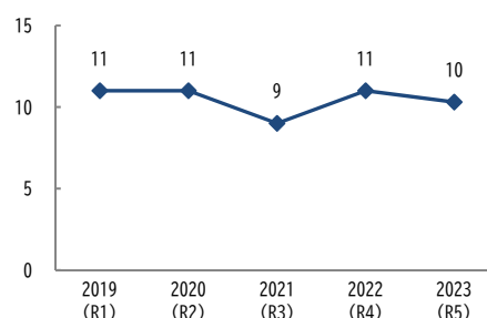
(ppmC) 非メタン炭化水素濃度の経年変化（2局平均値）
