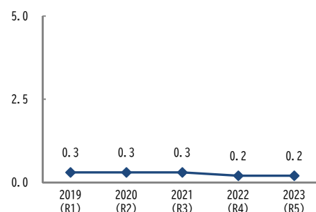
(mg/m³) 浮遊粒子状物質濃度の経年変化（全局平均値）
