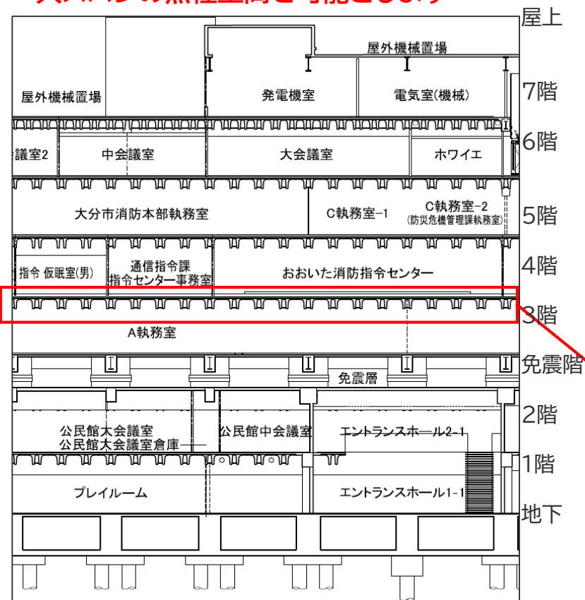
荷揚複合公共施設 断面図
