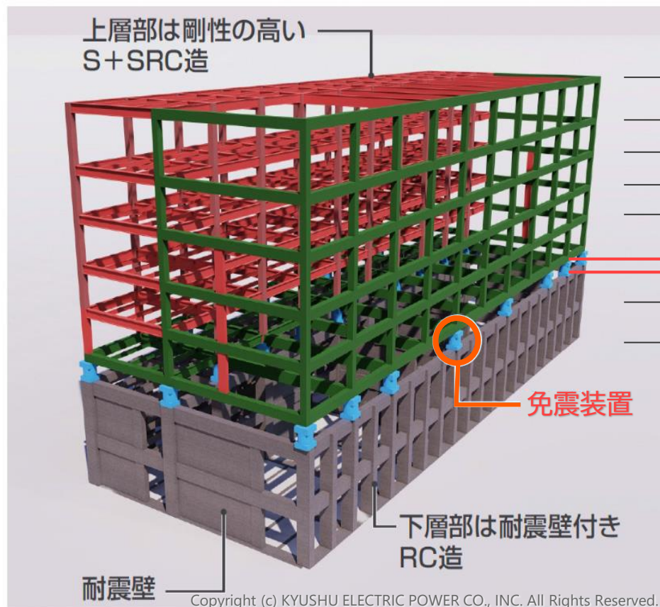
ハイブリッド構造の架構イメージ
