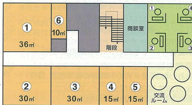
メインインキュベーション ブレインキュベーション [3階平面図]
