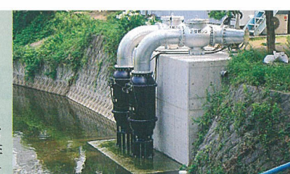
▲設置された災害対策ポンプ
