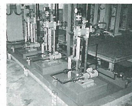
薬品注入ポンプ(横尾浄水場)
