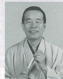
林家木久蔵
