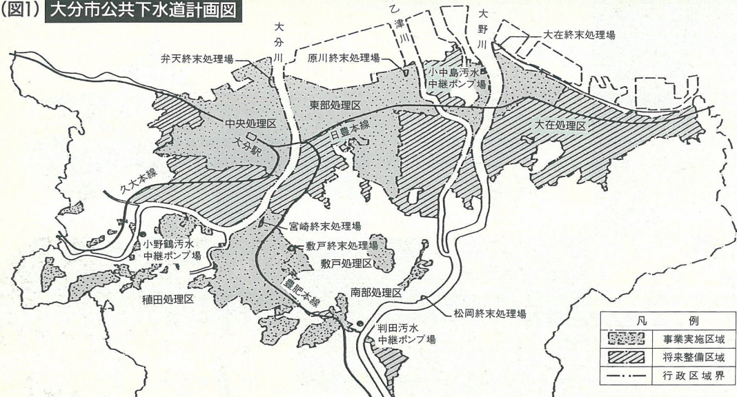
(図1) 大分市公共下水道計画図
