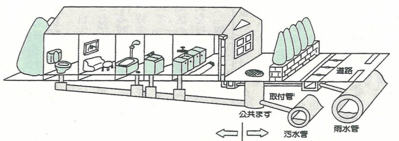
排水設備工事 (個人が工事費を負担し管理する) 公共下水道 (市が工事費を負担し管理する)
