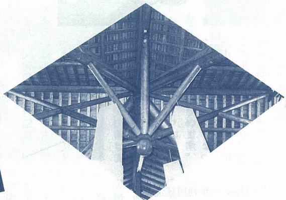
ホールの吹き抜けに見られる大屋根を支える傘構造（逆叉首構造）
