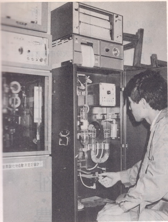
三佐小学校のオキシダント自動測定器
