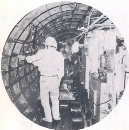
シールド工法による下水道工事
