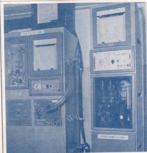
三佐小学校に設置された窒素酸化物自動測定器
