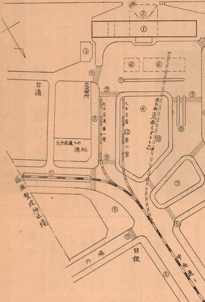
大分駅前広場施設設計平面図
