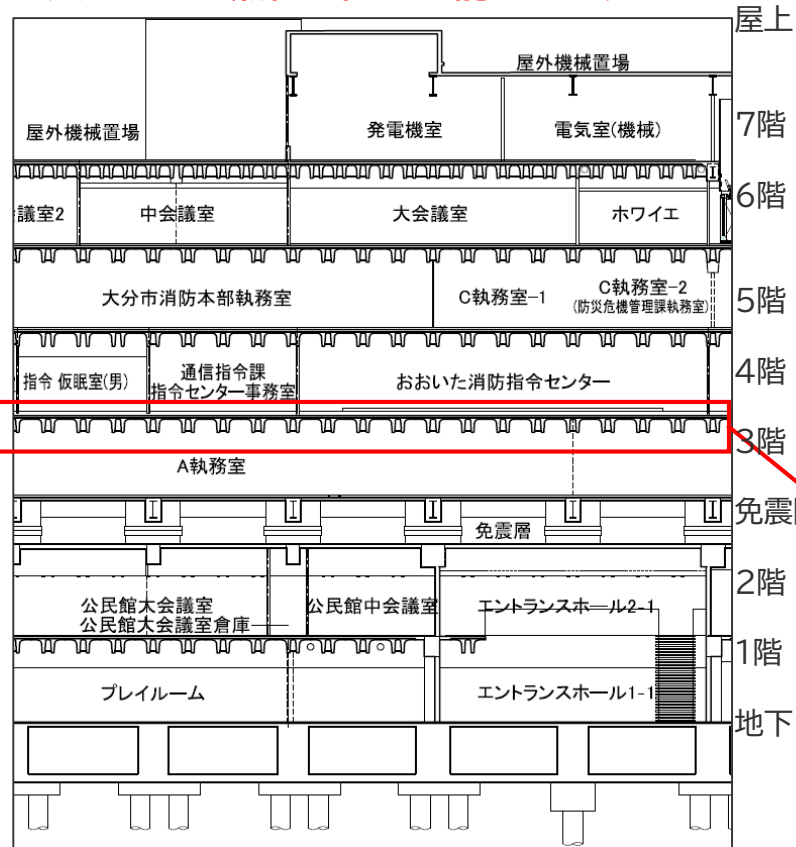
荷揚複合公共施設 断面図
