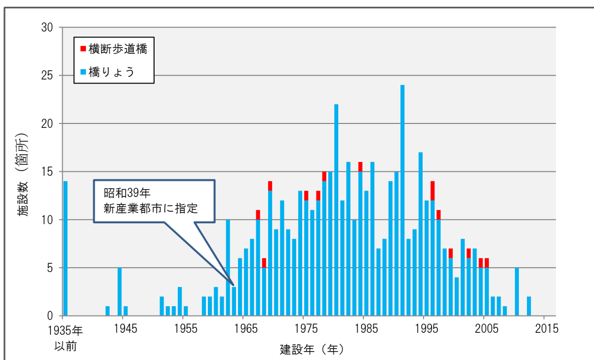
市管理橋りょう架設年度分布
