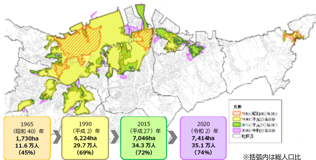
人口集中地区（D I D）の推移
