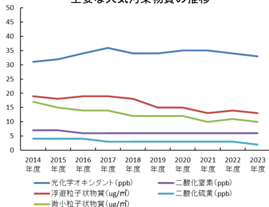
主要な大気汚染物質の推移
