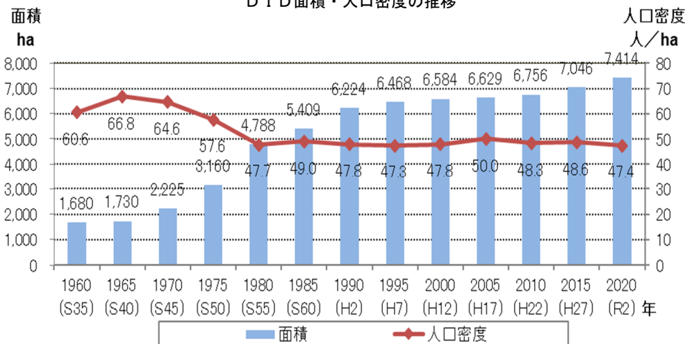
D I D面積・人口密度の推移
