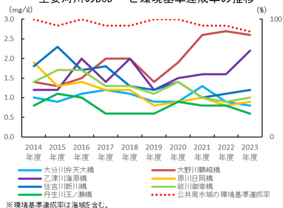
主要河川のBOD※ 3 と環境基準達成率の推移
