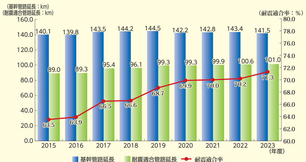
基幹管路の耐震適合率の推移
