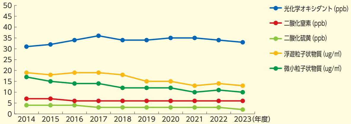
主要な大気汚染物質の推移
