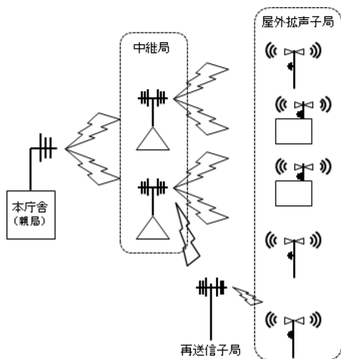
別表第 1 同報系防災行政無線局の構成
