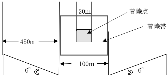
CH-47(最大55人乗)乗務員除く
