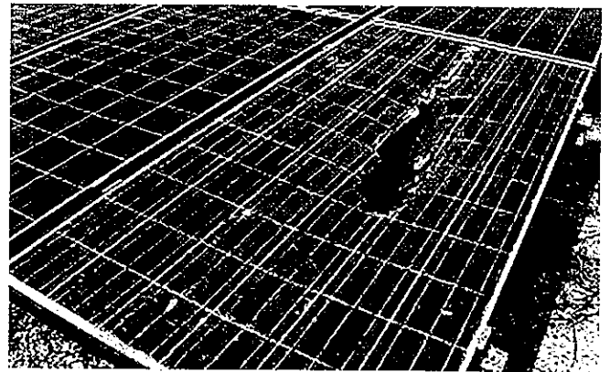
ホットスポットが原因となって発火した太陽光パネル
