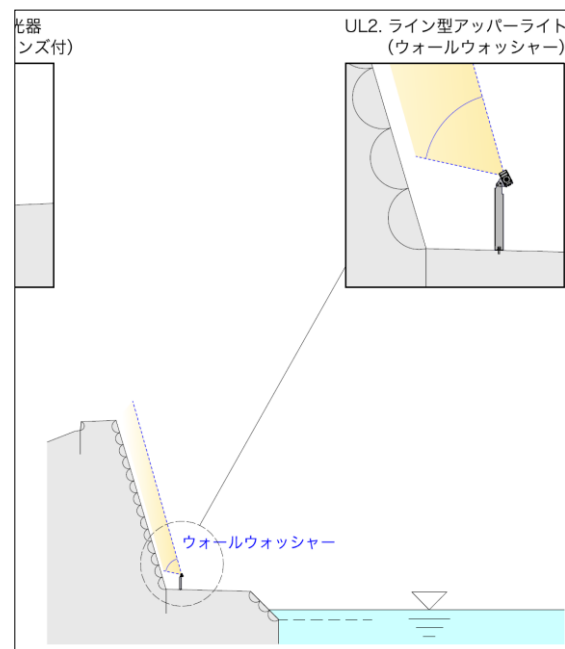
▲断面図(2)
