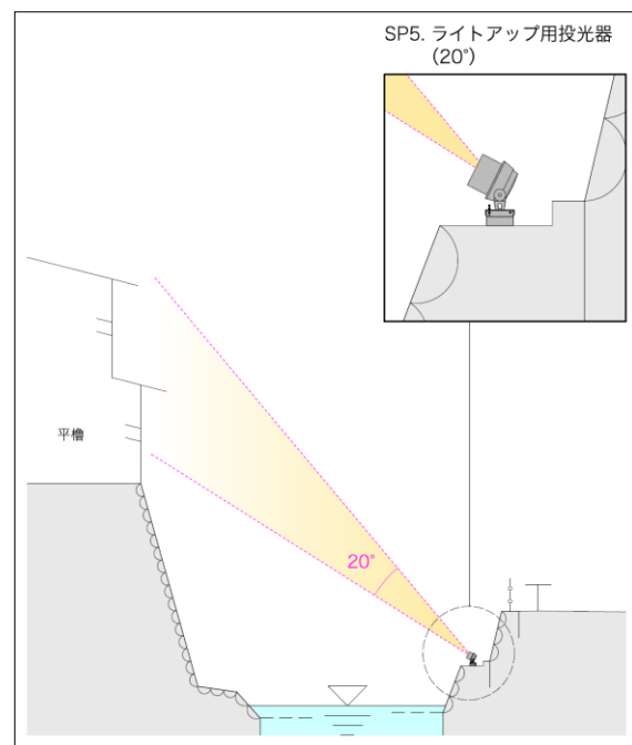
▲断面図(1)
