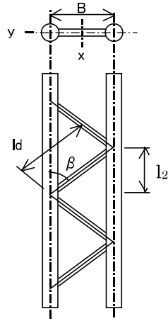
図-6.9 柱寸法図
