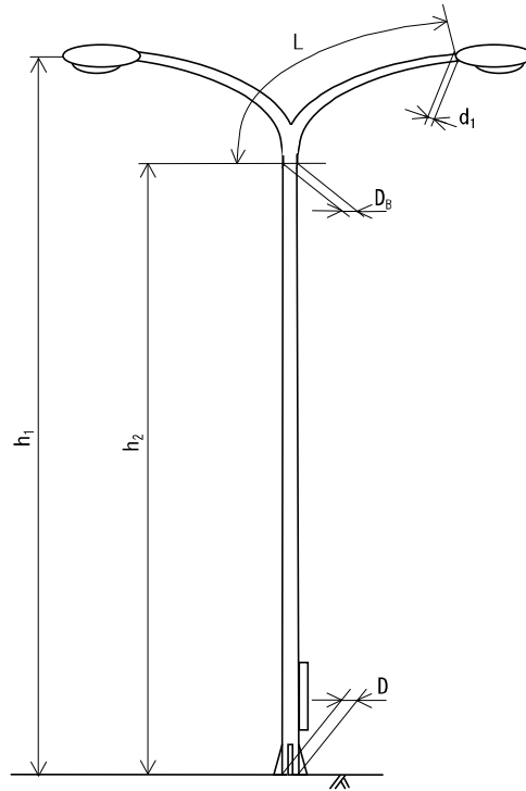
図-4. 1 照明ポールの形状寸法
