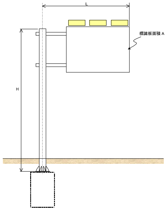
図－3. 1 F型標識柱の寸法図
