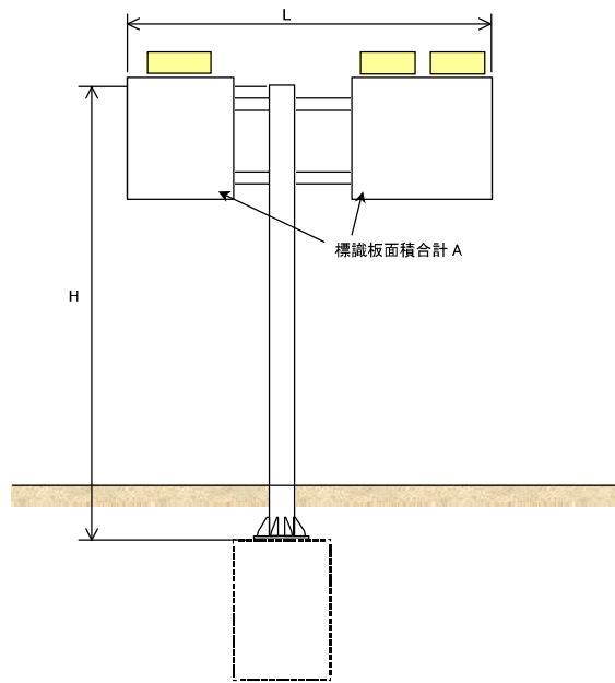
図-3.3 T型標識柱の寸法図
