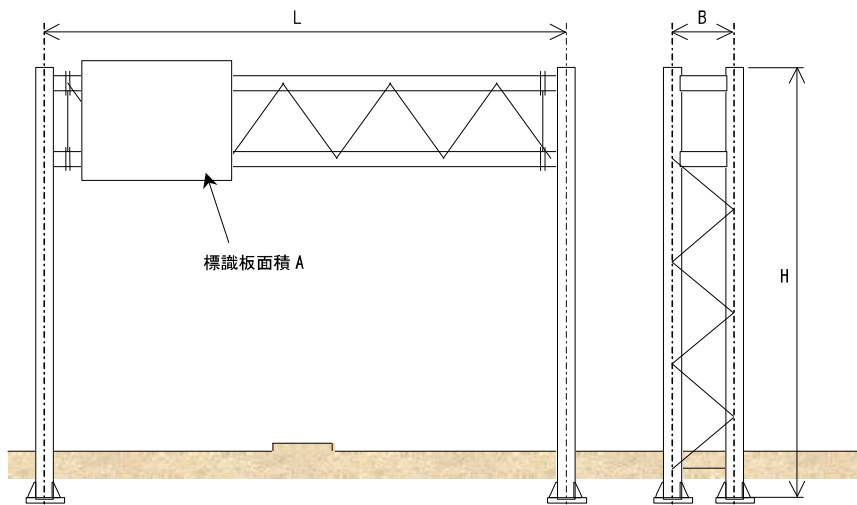
図-3.6 門型標識柱 (TYPE III) の寸法図
