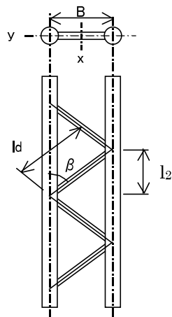
図-6.8 柱寸法図
