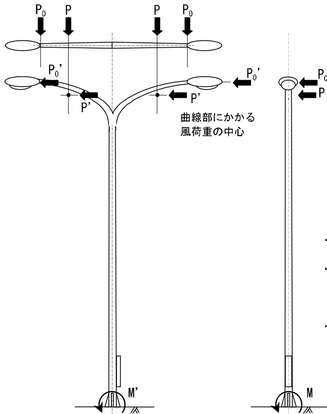
図一 4. 2 風荷重作用図
