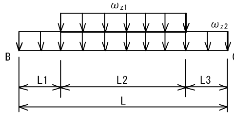
図-6.3 梁の荷重作用状態 (固定時)
