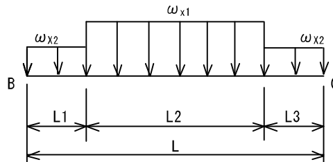
図-6.4 梁の荷重作用状態 (風時)
