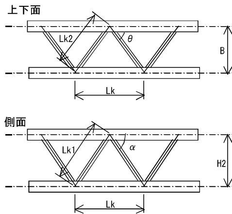
図一 6. 2 梁ヲス材の寸法図
