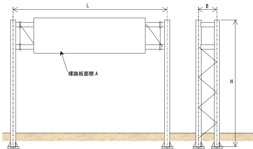
図-3.4 門型標識柱 (TYPE I) の寸法図
