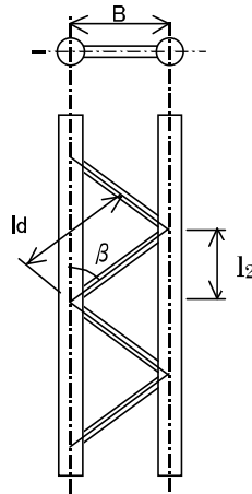
図-6.5 柱チラス材の寸法図
