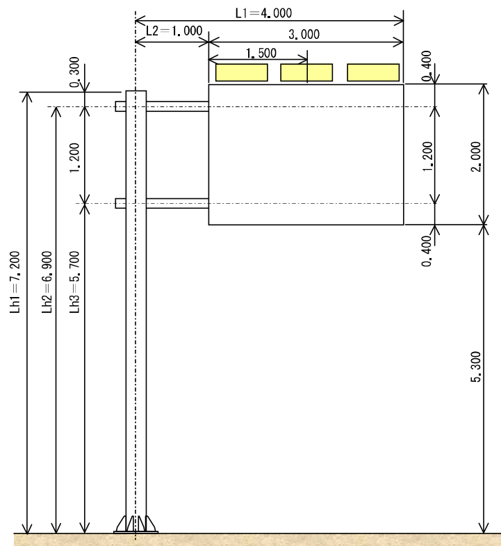
図－5. 1 形状寸法図
