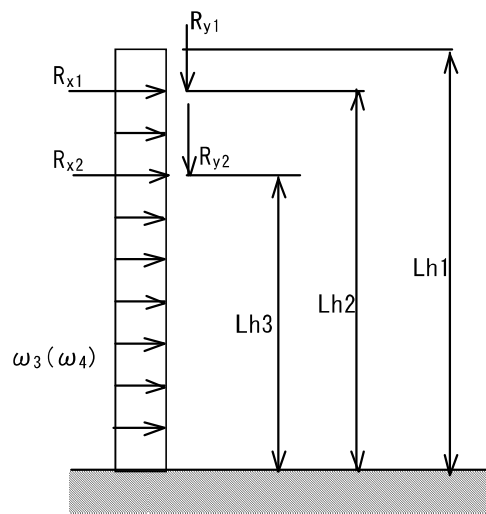
図-5.3 柱の荷重作用図
