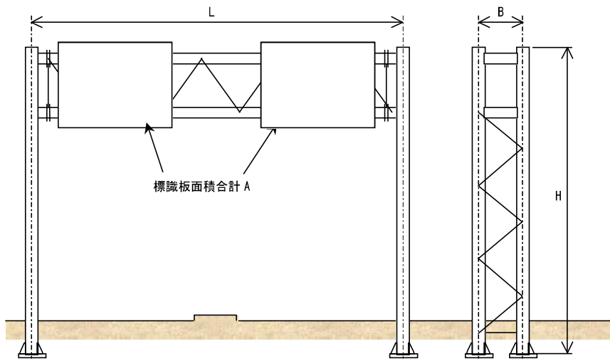
図-3.5 門型標識柱 (TYPE II) の寸法図
