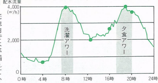
横尾浄水場配水流量経時変化
