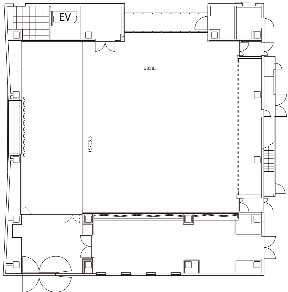
平戸間図
